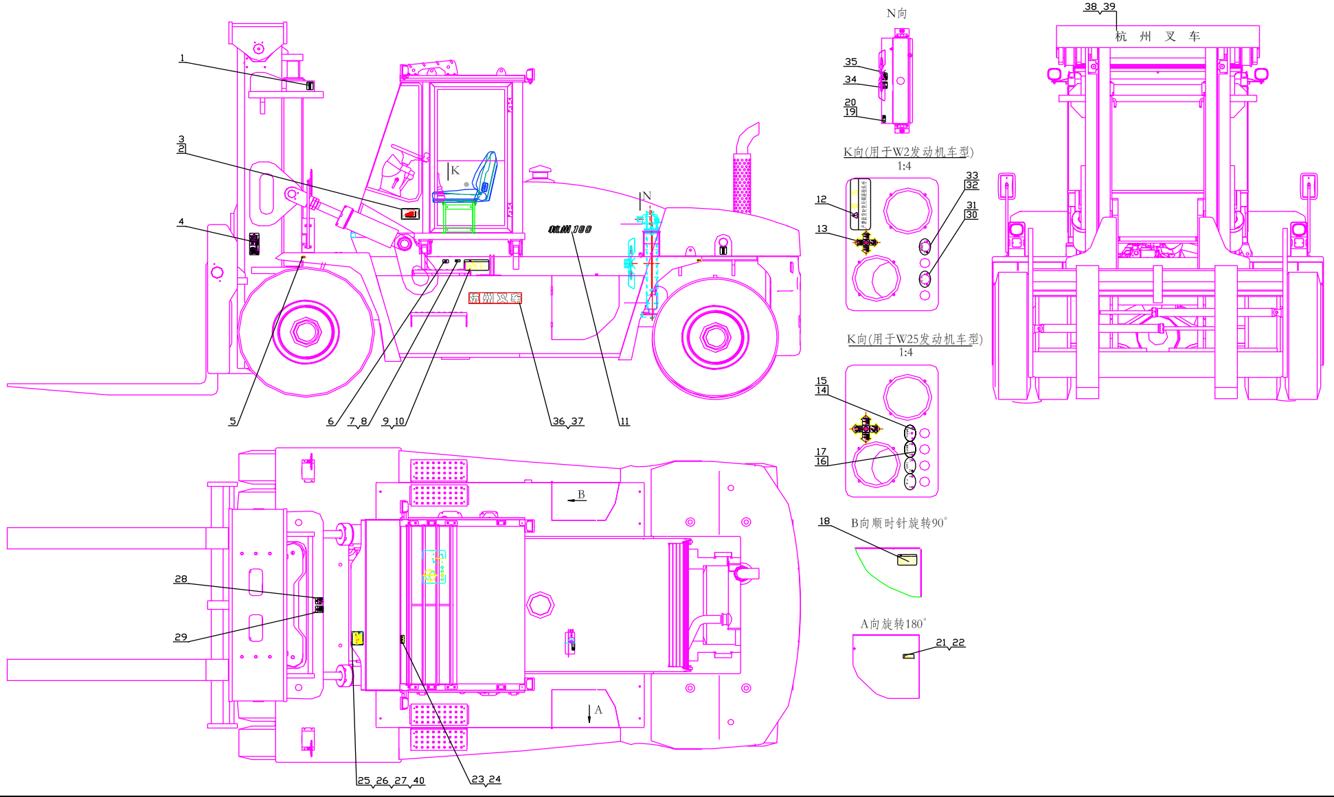
图1 标示 Fig.1 Nameplate
