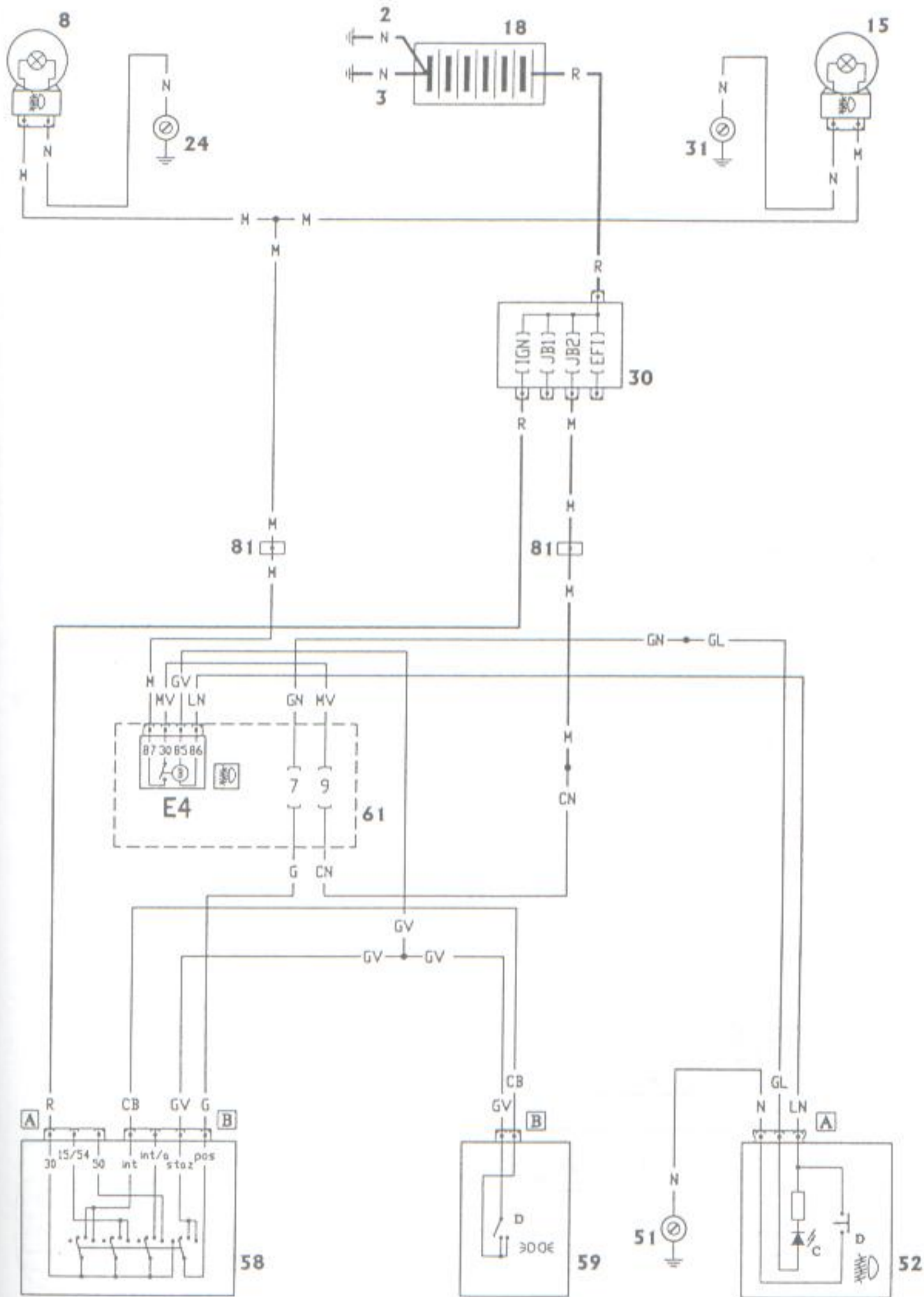
Rys. 10.3. Schemat połączeń przednich świateł przeciwmgłowych (objaśnienia oznaczeń cyfrowych i literowych w tekście)
